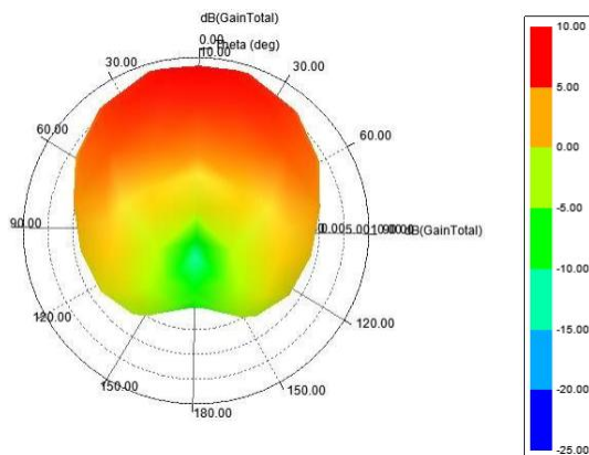
Fig. 8.Polar plot
